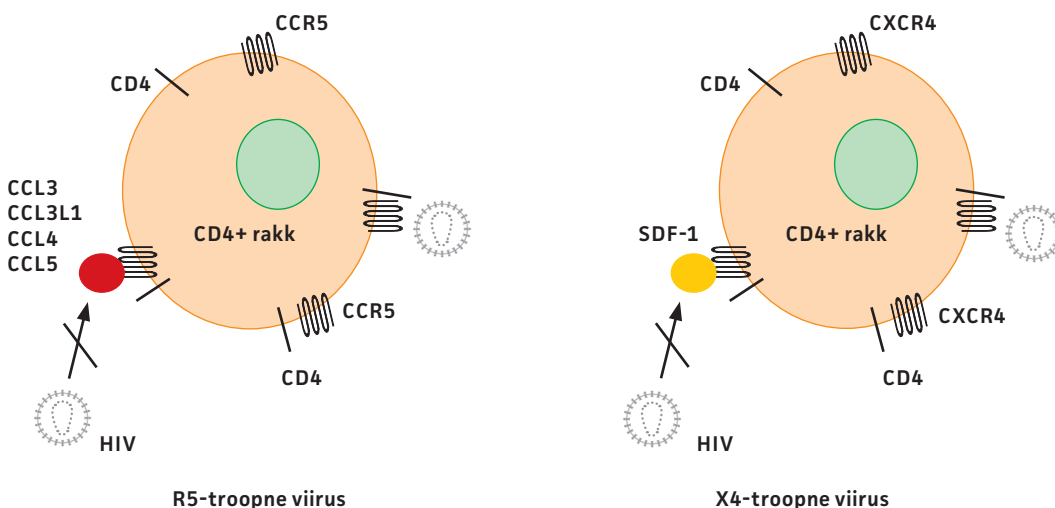
Joonis 3. Inimese immuunpuudulikkuse viiruse (HIV) koretseptorite kasutamine HIV ja peamiste naturaalselt R5- ja X4-troopsete viirused. CCR5 ligandid CCL3L1, CCL4 ja CCL5 (vasakul punasega) ning CXCR4 ligand SDF-1 (paremal kollasega) konkureerivad HIVga vastavalt CCR5 ja CXCR4 retseptoritele, blokeerides HIV sisenemist raku.
