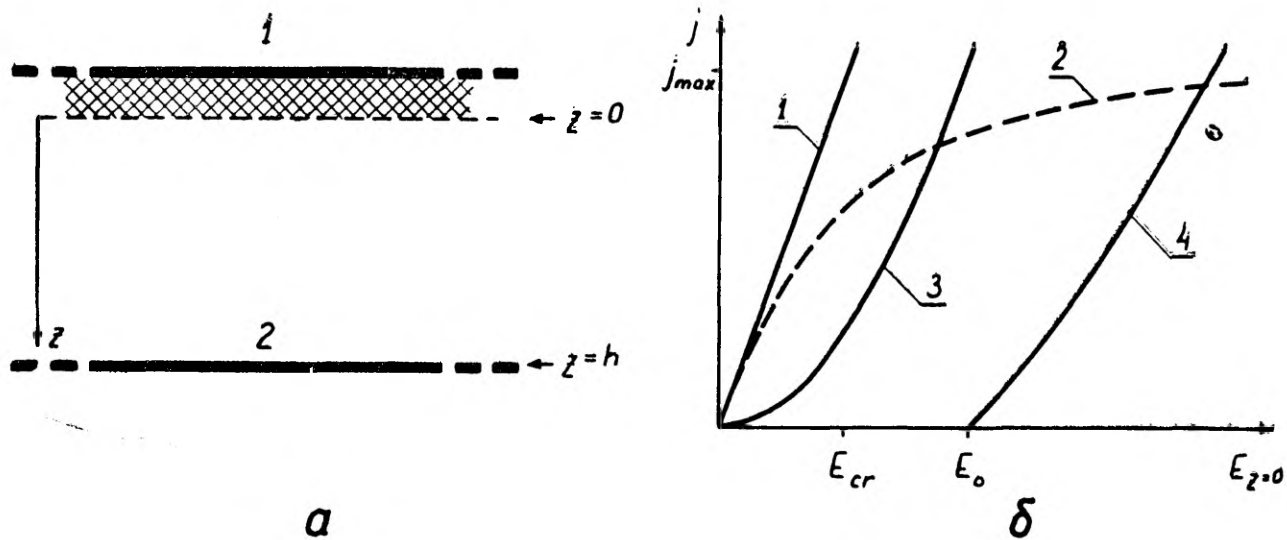
Рис. 1. a — схематизированный разрез нейтрализатора:
