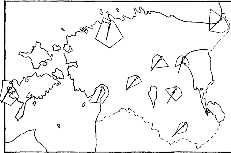
Joonis nr. 98. Keskised tuule teed jaanuaris 1923—35.
