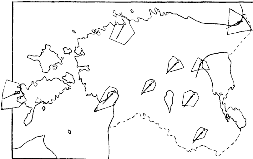
Joonis nr. 107. Keskmised tuule teed oktoobris 1923—35.
