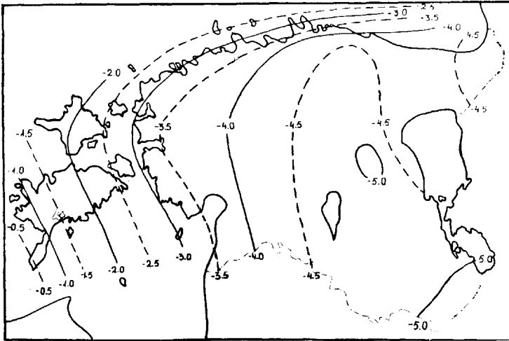
Joonis nr. 16. Detsembri isotermid.
