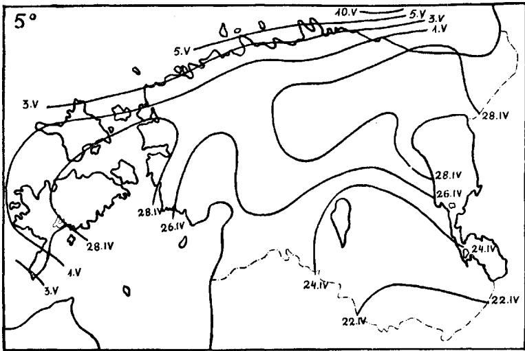
Joonis nr. 22. 5^{\circ} isotermi nihkumine kevadel.
