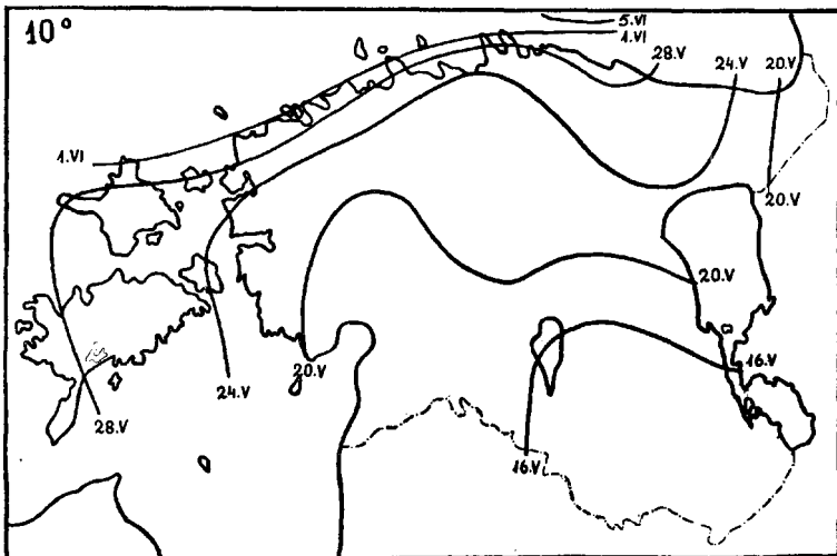
Joonis nr. 23. 10^{\circ} isotermi nihkumine kevadel.
