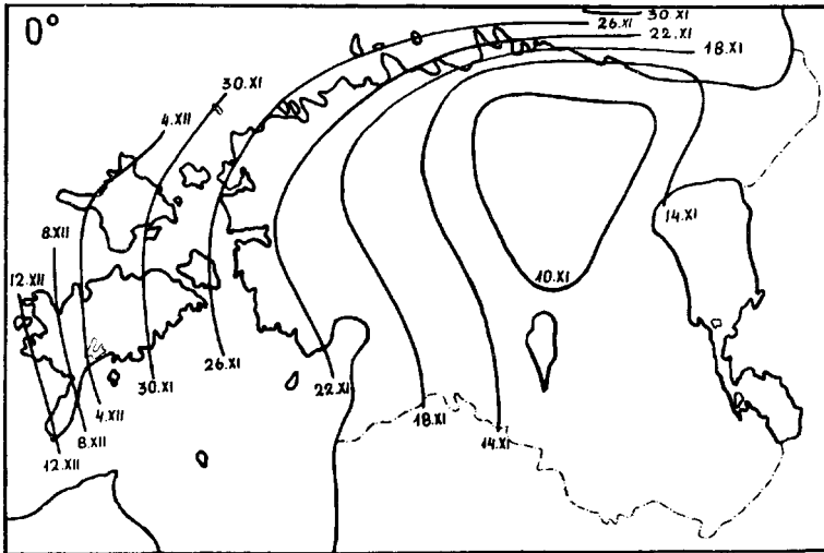
Joonis nr. 28. 0 o isotermi nihkumine sügisel.
