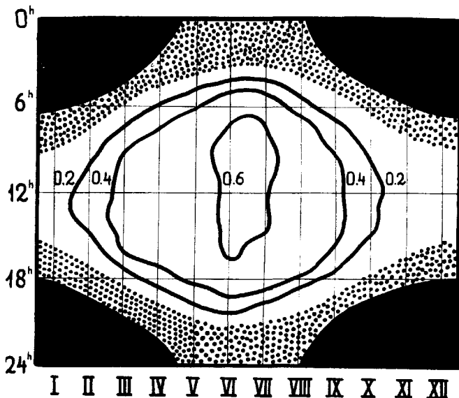
Joonis nr. 78. Päikesepaiste isopleedid Tallinnas 1923—35.
