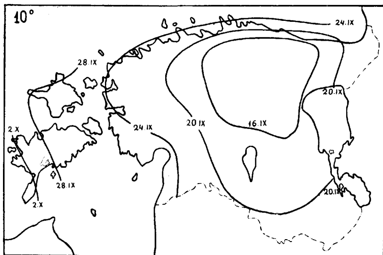
Joonis nr. 26. 10 0 isotermi nihkumine sügisel.
