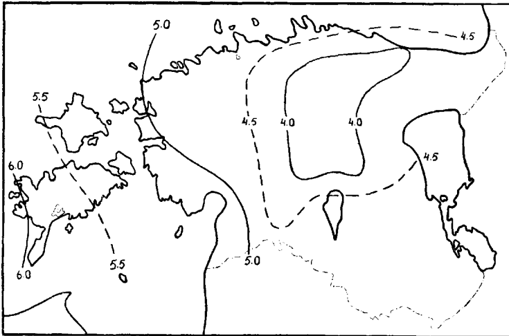
Joonis nr. 17. Aasta isotermid.
