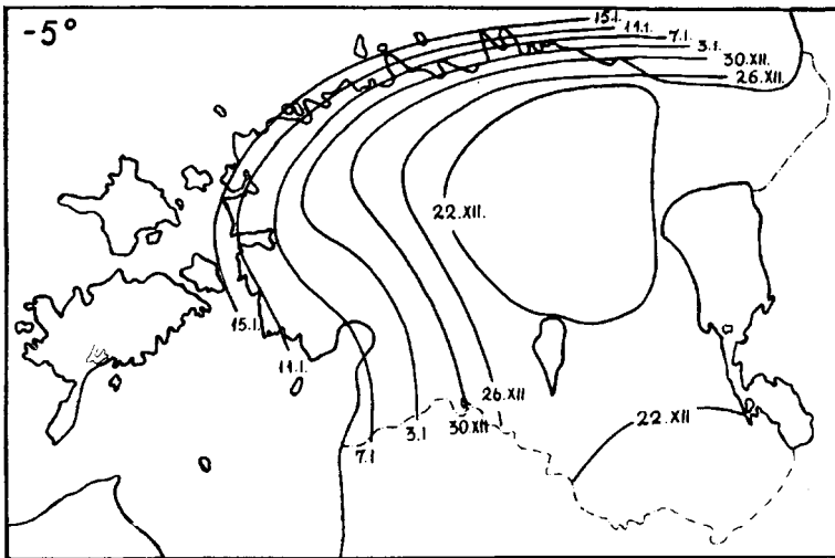
Joonis nr. 29. -5 o isotermi nihkumine talvel.
