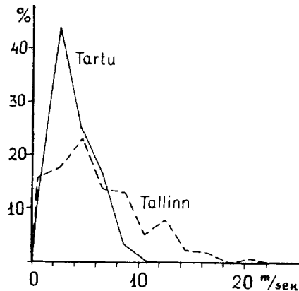
Joonis nr. 86. Tuule kiiruse sagedusjaotus Tartus ja Tallinnas veebruaris 1929—33.
