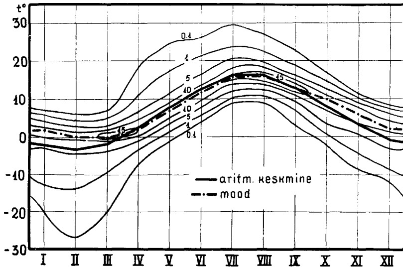
Joonis n r. 36. Õhutemperatuuride sageduste isopleetid protsentides vaatluste koguarvust Vilsandis 1923—37.
