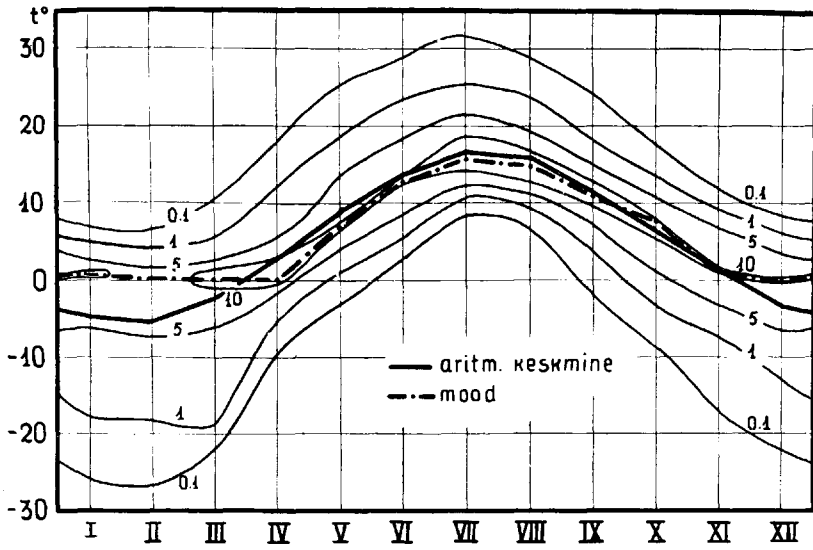
Joonis n r. 35. Õhutemperatuuride sageduste isopleetid protsentides vaatluste koguarvust Tallinnas 1923—37.
