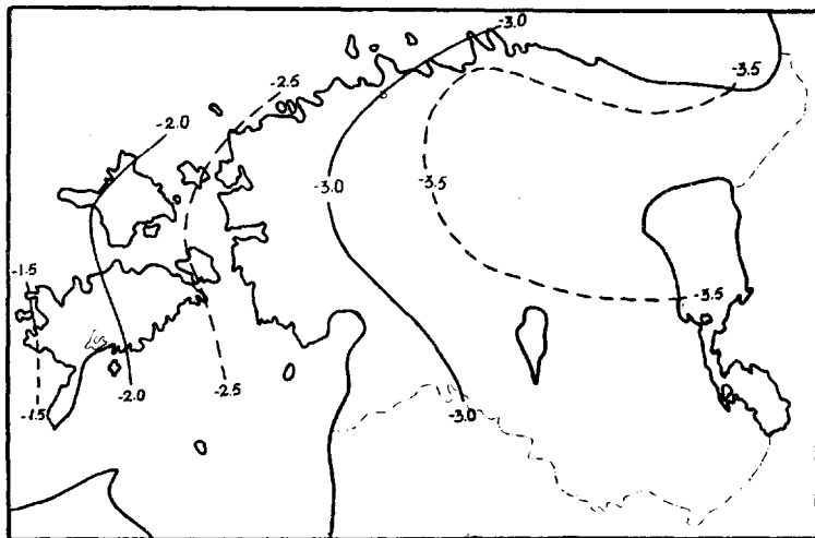
Joonis nr. 7. Märtsi isotermid.
