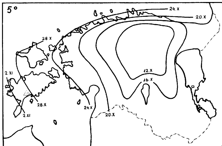
Joonis nr. 27. 5 0 isotermi nihkumine sügisel.
