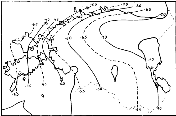
Joonis nr. 6. Veebruari isotermid.
