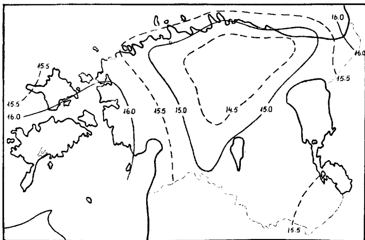
Joonis n. r. 12. Augusti isoterimid.
